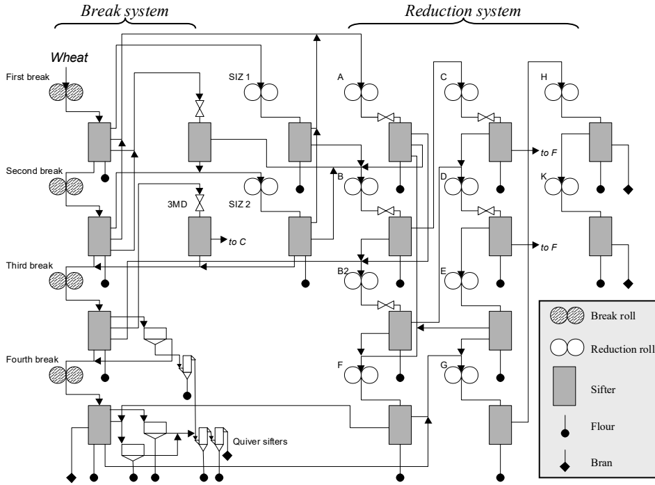
الشكل 19: مخطط نموذجي لمراحل لعملية الطحن
