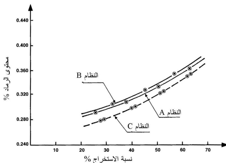
الشكل 7 منحنيات رماد تكاملية لأنظمة طحن مختلفة.
